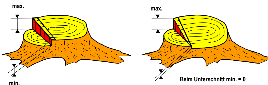
Abb. 15 Höhe der Bruchstufe (Minimum = 0 mm)
