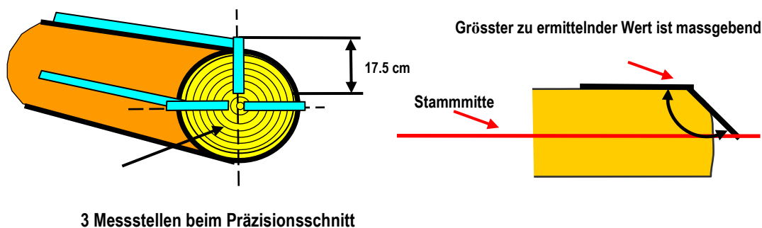
Abb. 35 Messstellen für die Winkelmessung bei geraden und bei schiefen Schnitten
