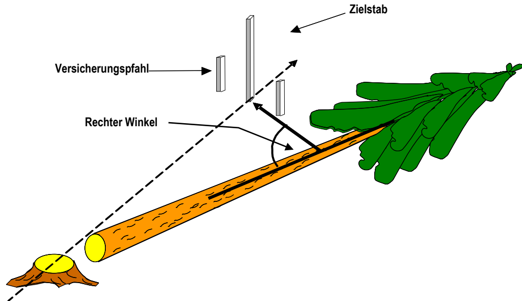
Abb. 10 Messung der Distanz rechtwinklig zum gefälltten Baum / Masten
