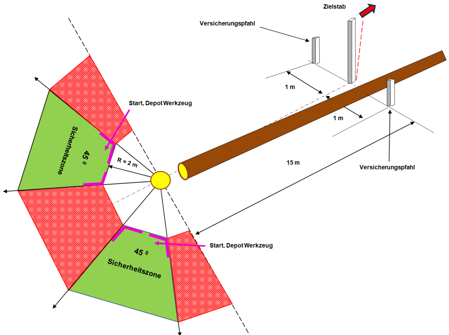
Abb. C Masten - Zielfällung
