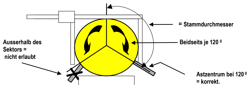
Abb. 38a Der Entastungssektor links und rechts 120 ° (entspricht dem Stammdurchmesser)
