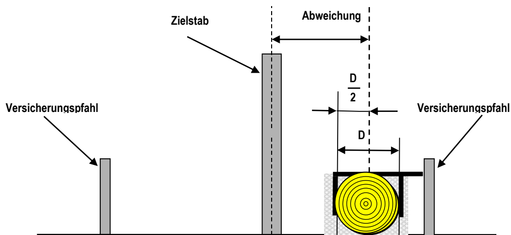
Abb. 11 Abweichung von der Fällrichtung
