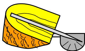
Abb. 13 Messen der Fallkerbe bei geraden und bei runden Schnitten
