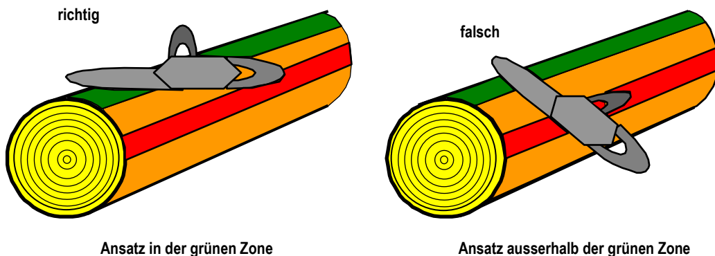
Abb. 29 Ansatz der Motorsäge beim Abwärtsschnitt in der grünen Zone
